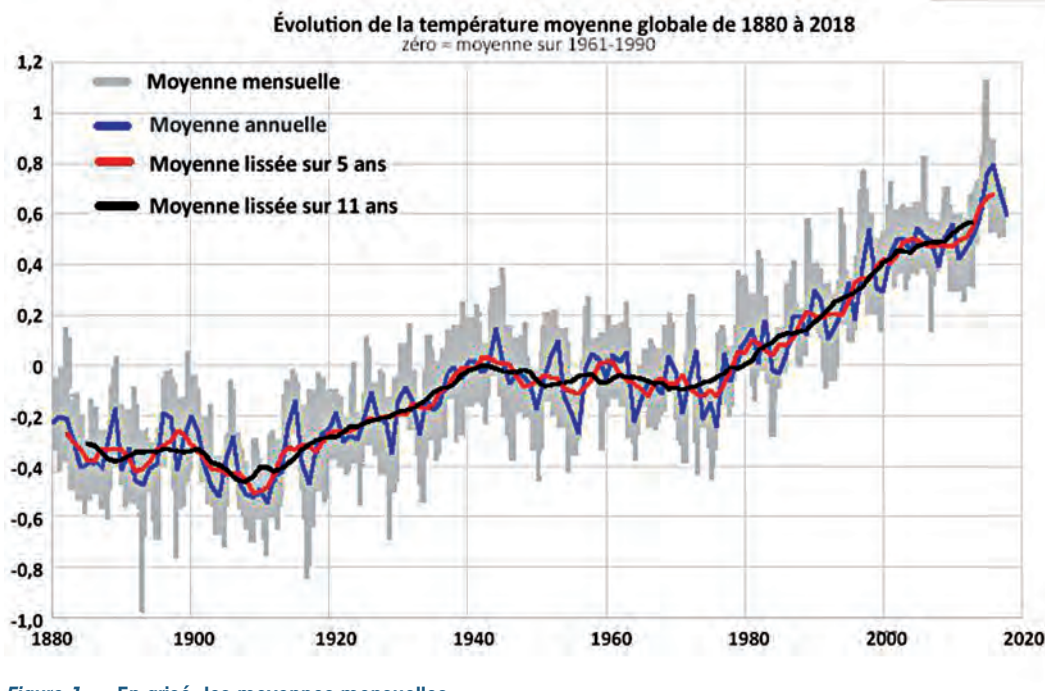
Figure 1. — En grisé, les moyennes mensuelles; en bleu les moyennes annuelles, en rouge les moyennes glissantes sur 5 ans; en noir les moyennes glissantes sur 11 ans. L'ordonnée correspond à l'écart par rapport à la moyenne des années 1961-1990. Source : HadCRUT4 ( https://crudata.uea.ac.uk/cru/data/temperature/ ).
