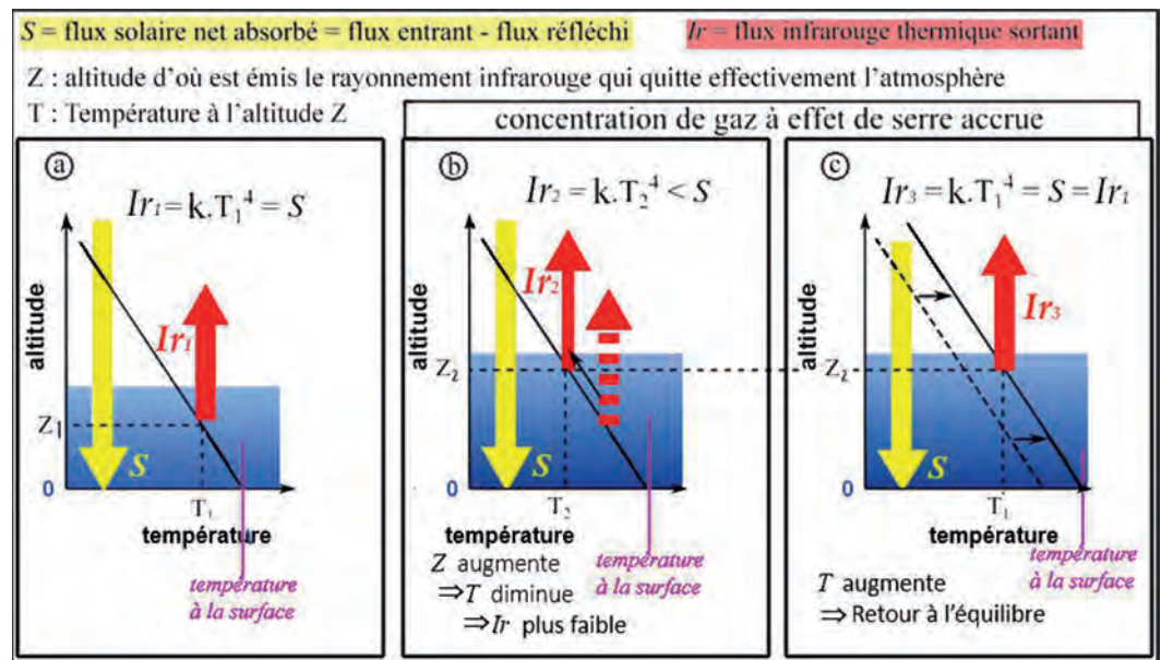
Figure 3. – L'augmentation de la concentration atmosphérique de gaz à effet de serre fait augmenter la température. La figure a montre le système dans son état initial, où l'énergie sortante équilibre l'énergie entrante. La ligne oblique schématise le profil vertical de température de la troposphère, dont la pente est fixée par la thermodynamique. Si la concentration de gaz à effet de serre croît (figure b), les infrarouges qui peuvent quitter l'atmosphère n'emportent plus assez d'énergie. La température de l'atmosphère doit croître pour que le système atteigne un nouvel équilibre (figure c), et, la pente du profil vertical étant inchangée, la température croît simultanément au niveau de la surface. (Des explications détaillées peuvent être trouvées dans un article de Jean-Louis Dufresne et Jacques Treiner paru dans la Météorologie en février 2011.)
