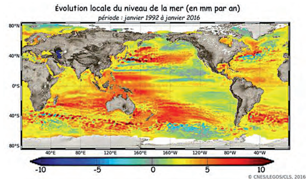
Figure 4. – Le niveau de la mer ne monte pas de façon uniforme. Certaines régions, telles que les États insulaires du Pacifique, subissent une élévation 10 fois plus rapide que d'autres régions.
